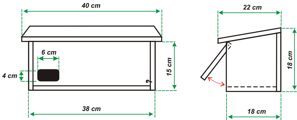
Rys. 2. Schemat budowy drewnianej skrzynki dla jerzyka
