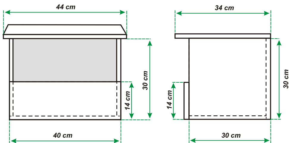
Rys. 3 Schemat skrzynki lęgowej dla pustulek
